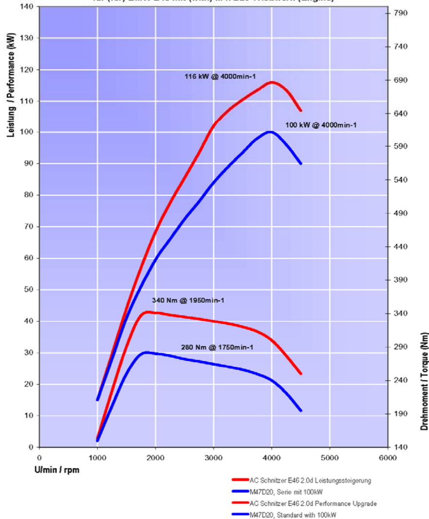
AC Schnitzer Leistungssteigerung (Performance Upgrade) für (for) BMW E46 mit (with) M47D20 Triebwerk (Engine)
