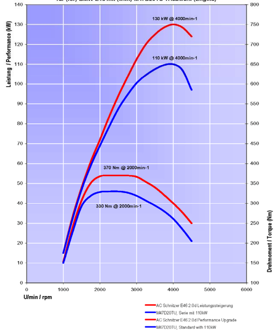
AC Schnitzer Leistungssteigerung (Performance Upgrade) für (for) BMW E46 mit (with) M47D20TU Triebwerk (Engine)
